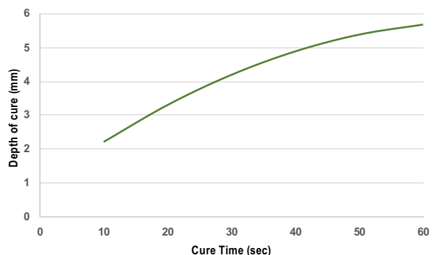
Profondità indurimento (50 sec, 250 mW/cm 2 , 405nm) mm 5 – 6
